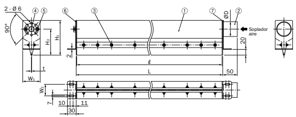
① Cuerpo ② Tubo de entrada ③ Tornillo de ajuste (M4) ④ Tornillo (M10) ⑤ Tornillo (M5) ⑥ ⑦ Soporte
